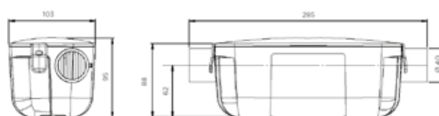
Dimensões (mm)
