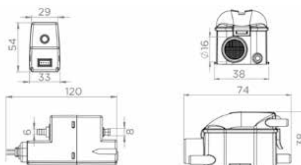
Dimensões (mm)
