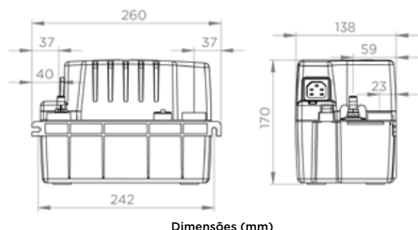
Dimensões (mm)
